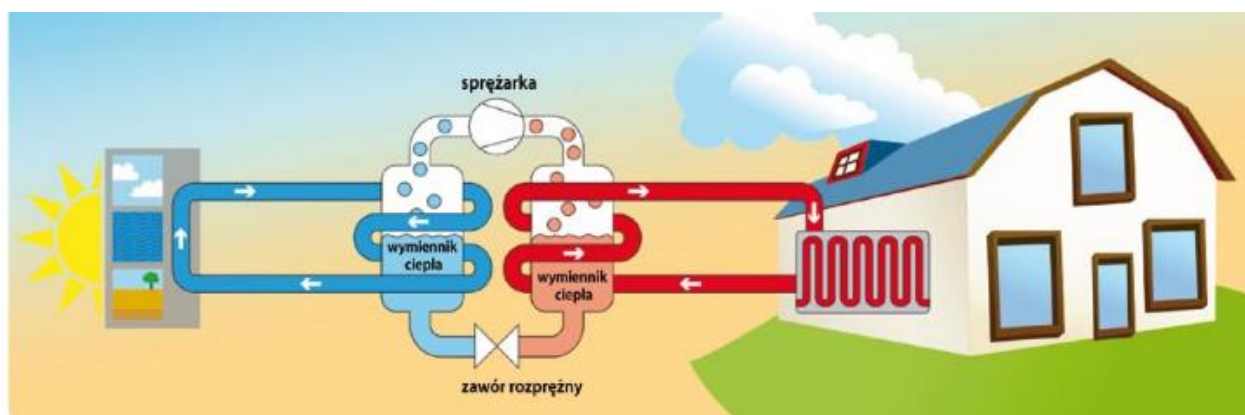
Rysunek nr 4.5-4. Schemat działania transformatora ciepła
