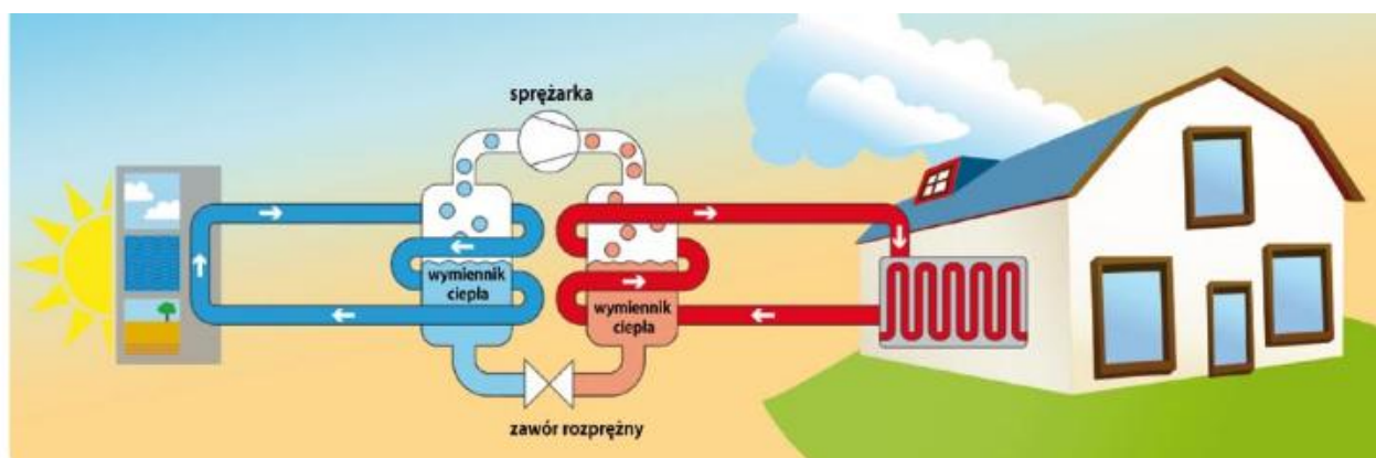
Rysunek nr 4.5-4. Schemat działania transformatora ciepła
