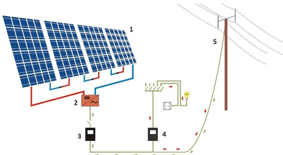
Rysunek nr 4.5-2. Uproszczony schemat instalacji PV podłączonej do sieci energetycznej
