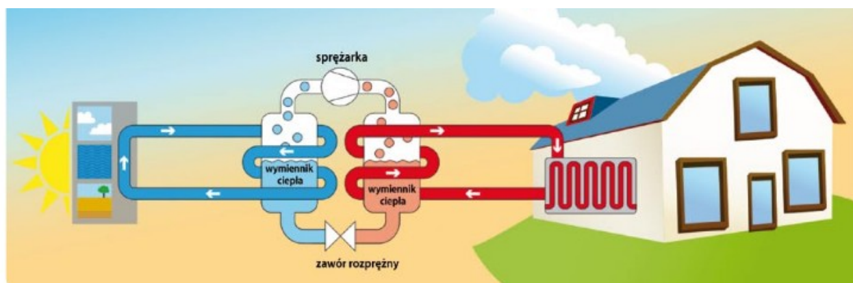
Rysunek nr 2.18-4. Schemat działania transformatora ciepła
