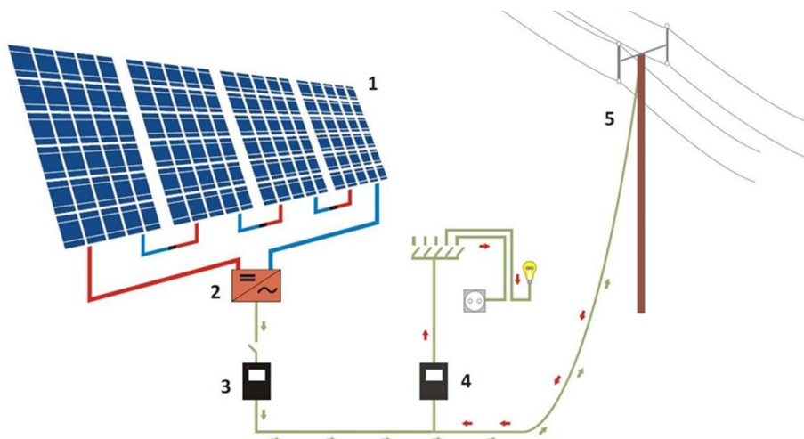
Rysunek nr 2.18-2. Uproszczony schemat instalacji PV podłączonej do sieci energetycznej
