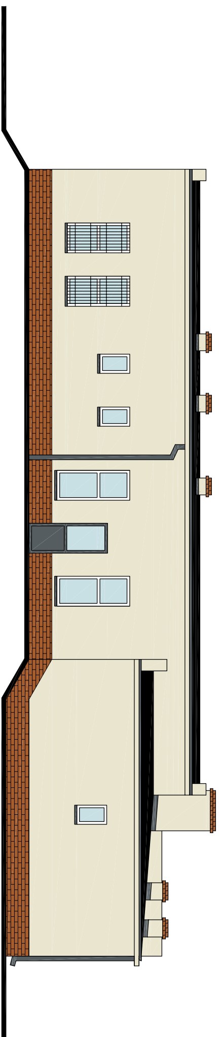
ELEWACJA POŁUDNIOWA 1:100
