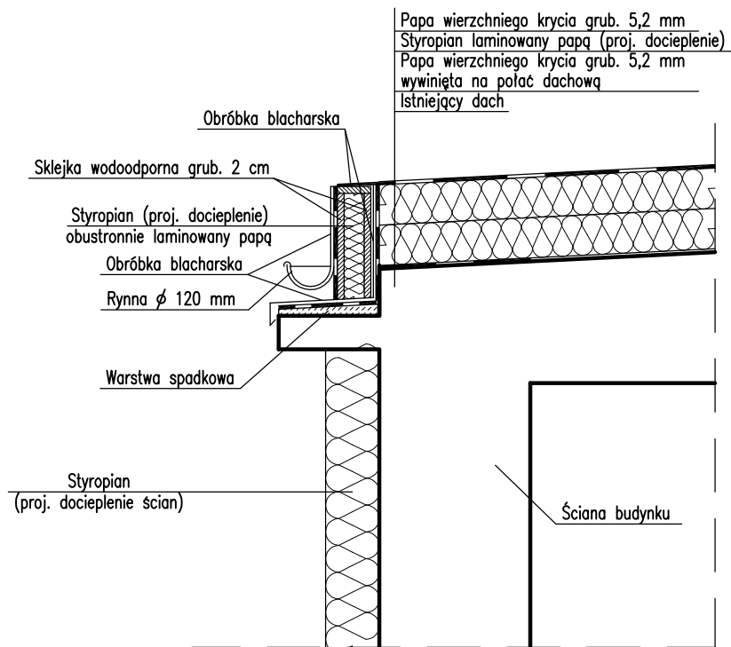
Rynny dachowe, rury spustowe i obróbki blacharskie z blachy stal. powlekanej poliestrem mat. RAL 7011
