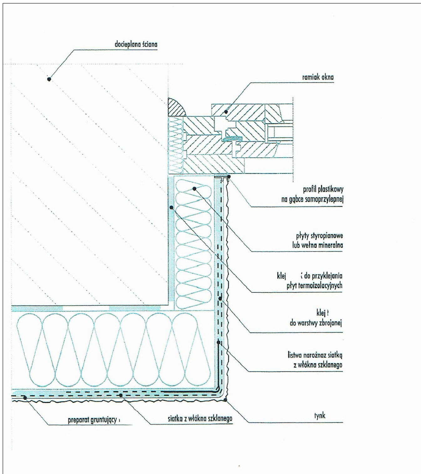
Detal docieplenia ościeża okiennego lub drzwiowego
